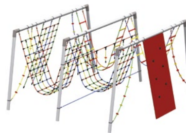
PD-4587-10 Erda Alapterület: 5,5x5,3 m Területigény: 8,6x8,9 m Esésmagasság: 2,7 m
