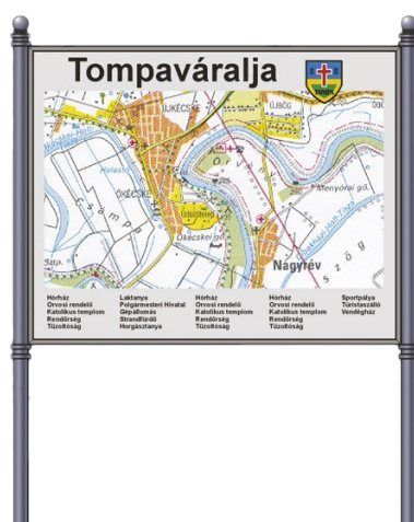
IT-21 Közepes méretű térképes infotábla Egyoldalas színes térképpel, felirattal ellátva színterezett acélcső oszlop Ø 60 mm Szélesség: 1500 mm Magasság: 2000 mm Táblaméret: 1500 x 1200 mm Lebetonozható kivitelben.
