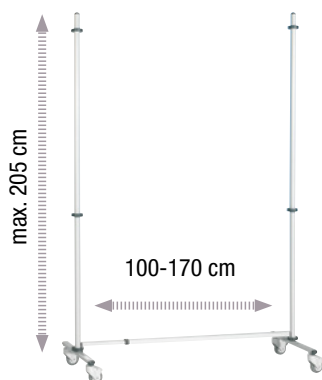
T-ÁLV-G görgős T-állvány
