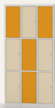
FITTMET-30 5003-9-500-ST 9 rekeszes 90 x 180 x 50 cm
