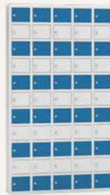
LockMet / WSS 55 55 rekeszes / 93 x 168 x 20 cm
