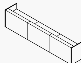
AS-REC-OL-80 2 db Javasolt asztalméret: AS-REC-EL-160 3 db 3 db 160 x 80 cm-es asztal 484 x 80 x 122 cm
