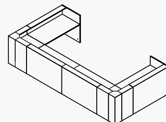
AS-REC-OL-80 2 db Javasolt asztalméret: AS-REC-EL-180 2 db 2 db 200 x 80-es, és AS-REC-SE-30 2 db 2 db 140 x 80 cm-es asztal AS-REC-EL-80 2 db AS-REC-EL-140 2 db 202/362/202 x 80 x 122 cm
